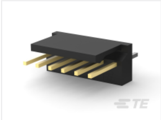
TE 产品编号 3-647078-6 06P MTA100 HDR HT FL 15AU LF
