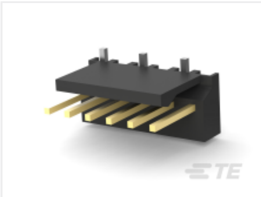
TE 产品编号 3-647167-6 06P MTA100 HDR ASSY SM 15AU LF
