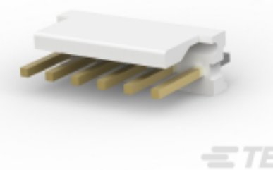
TE 产品编号 3-641119-6 06P MTA156 HDR ASSY FL/ST LF
