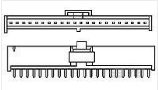
TE 产品编号1-1888291-9 FPH-1321G=FLXPAC HDR P 13 ST LF
