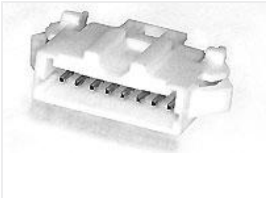
TE 产品编号1-292215-6 MINI CT SGL RELAY 16P NAT
