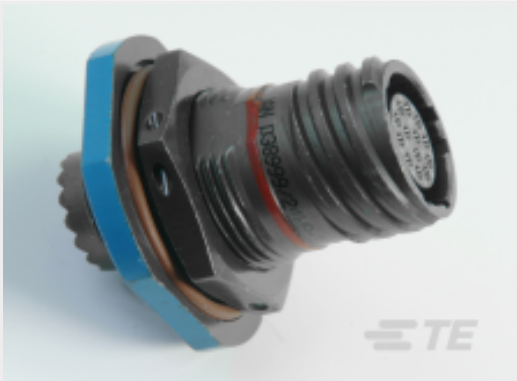
TE 产品编号YDTS24T15-18PNV001 RECP ASSY
