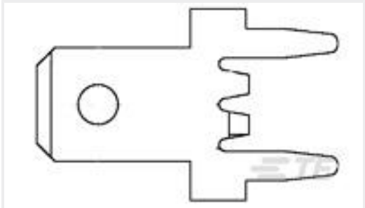
TE 产品编号63823-1 187 FASTON TAB TPBR
