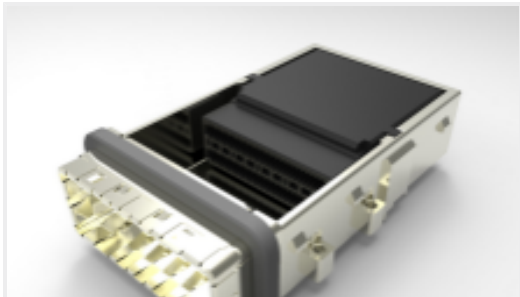
TE 产品编号CAT-C3106-C76264 CDFP 壳体组件
