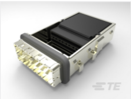
TE 产品编号 CAT-C3106-C76264 CDFP 壳体组件
