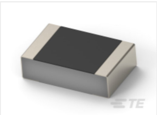
TE 产品编号8-2176452-9 CPF 0201 4K42 0.1% 25ppm 1K RL
