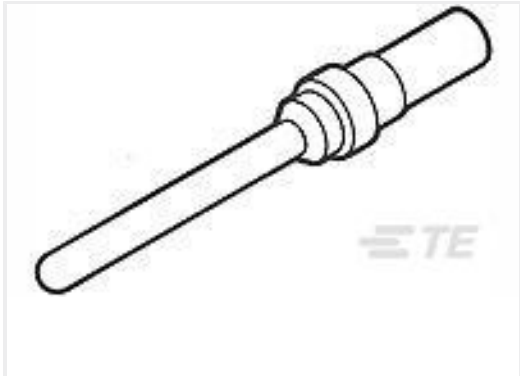
TE 产品编号205089-1 HD 20 PIN CONTACT
