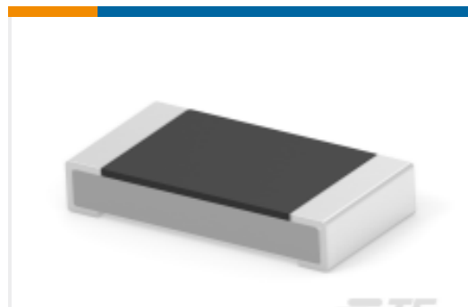
TE 产品编号4-2176392-9 RQ 1206 422K 0.1% 10PPM 5K RL
