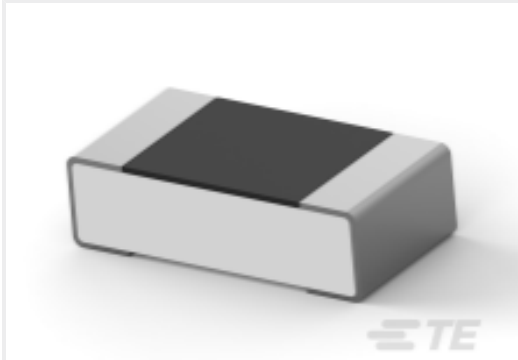
TE 产品编号3-2176372-6 RQ 0603 115K 0.1% 10PPM 5K RL
