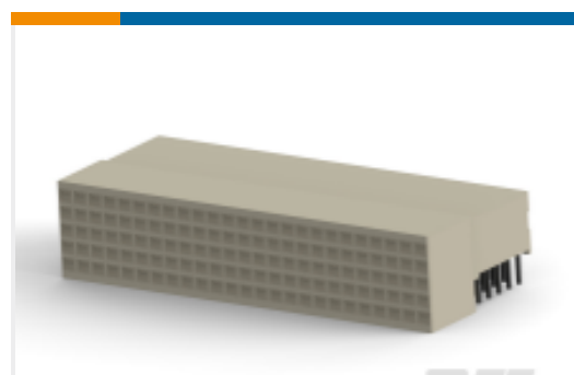
TE 产品编号5646487-1 HM 插座连接器：传统背板，共面，2mm
