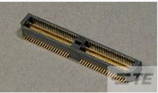
TE 产品编号 3-1658463-2 MSB0.80PL5ASY56DP,GP,30,VCTY
