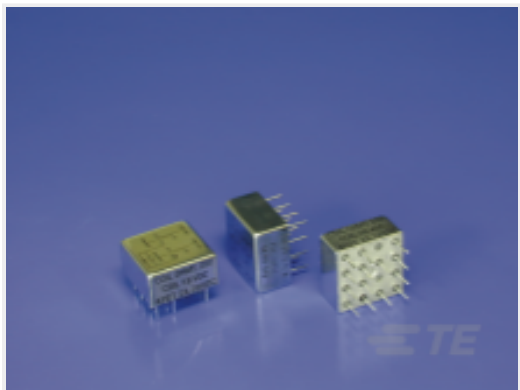
TE 产品编号 1-1617076-1 3SBH1139A2 = M39016/14-002M
