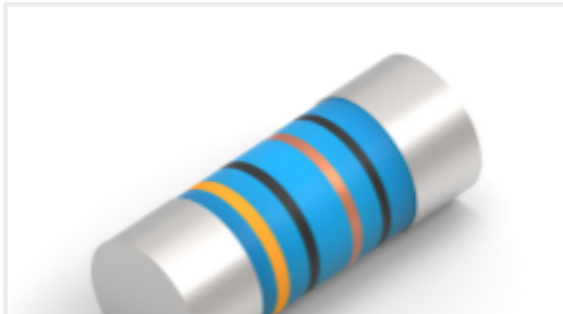
TE 产品编号7-2176316-2 MELF SMA_A 68K 1% 50PPM 0207 1W
