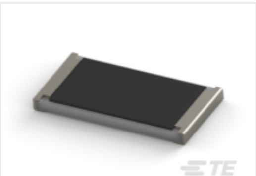
TE 产品编号CAT-C339-A76A SMD 功率电阻器：2 瓦特，3521 系列
