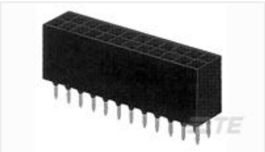
TE 产品编号1-534236-5 30 MODII VRT DR CE 100/120
