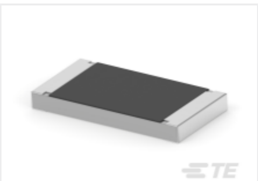
TE 产品编号1-2176350-1 CRGCQ 2512 47R 5%
