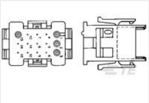
TE 产品编号1-640514-0 20P MR II CAP HSG V0
