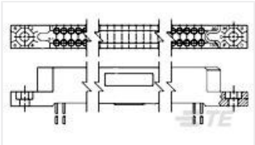
TE 产品编号202844-5 BOX RECP 30 POS STAG
