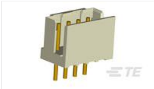
TE 产品编号292134-5 CT BOX HDR ASSY V 5P AU W/KINK
