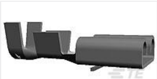
TE 产品编号42281-1 FF 250 REC 18-14AWG BR
