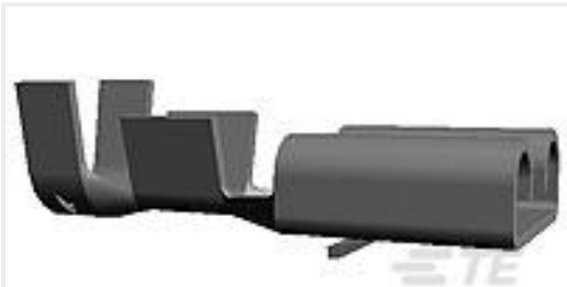
TE 产品编号60249-1 FF 250 REC 16-12AWG BR
