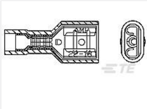
TE 产品编号735278 EPEZT * STECKHUELSE ISOLIERT 6,3 X 1,0 *
