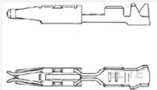
TE 产品编号929952-1 MT1 REC 1.6 Contact SRC Sn
