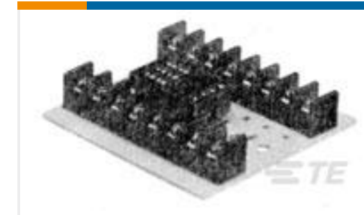
TE 产品编号 1393837-1 27E460=SOCKET,R10,2POLE,TRACK- MNT,SCREW
