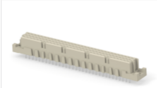
TE 产品编号224411-E STVC 64 F AC VV 7-00 TL 4,0 * 247 E007 1
