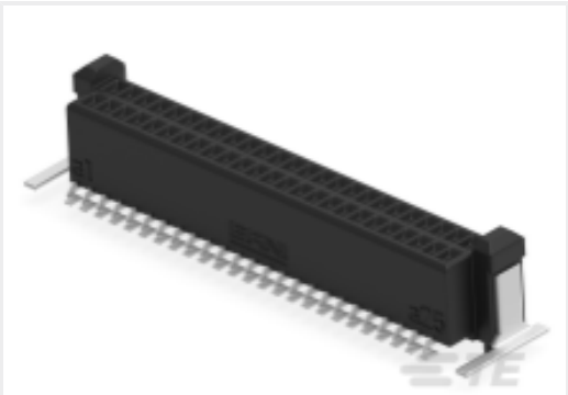
TE 产品编号294006-E DRCB 0,80 50 F SMD F4 137 E009 094 GU-H
