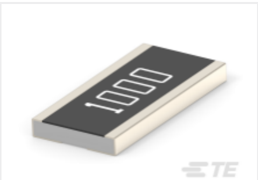
TE 产品编号9-2176566-9 3430 A3 1% 11K 100ppm 1k RL
