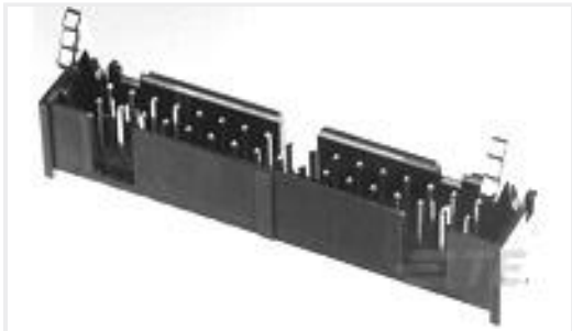
TE 产品编号2-1761608-3 IDC LOW PRO HDR 10P VERT SHT L
