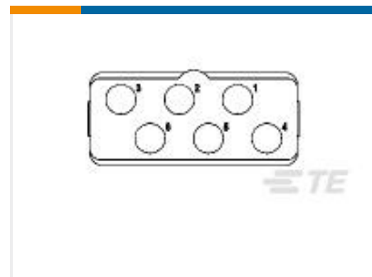
TE 产品编号1738101-1 Insert Asy,Pin,Arr 06,Environ,Key B
