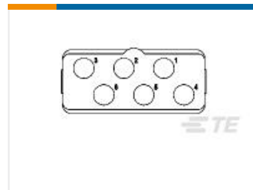
TE 产品编号1738099-1 Insert Asy,Socket,Arr 06,Environ,Key A
