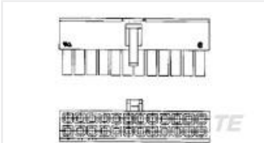
TE 产品编号1586075-4 4P RCPT VAL-U-LOK V2 BLK
