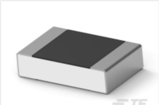
TE 产品编号9-2176373-7 RQ 0805 100R 0.1% 10PPM 1K RL
