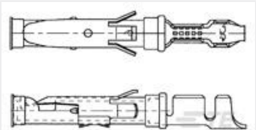
TE 产品编号1198133001 44A0221-16-4/8
