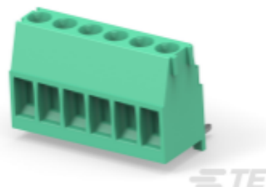
TE 产品编号 284414-6 TERMI-BLOK 900 PCB 6 POS 3,5 m
