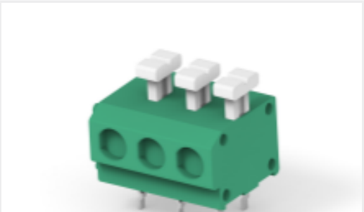
TE 产品编号1-2834018-3 3POS 5.0MM TEPS CONN.
