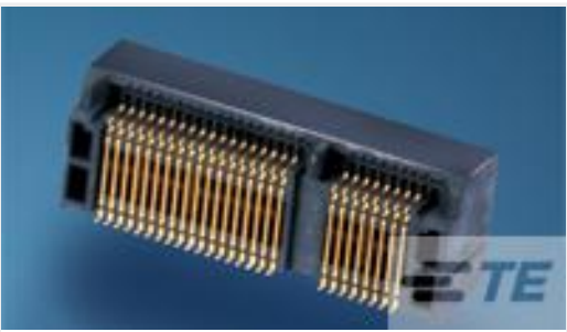
TE 产品编号1759546-1 0.8mm Mini PCI-Express 9.9 Height
