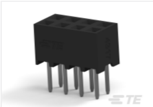
TE 产品编号 2314825-8 8P,2MM,B-B,REC,DRVT,2.7,0.38AU,TB,W/CAP
