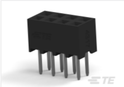
TE 产品编号 2314821-8 8P,2MM,B-B,REC,DRVT,2.7,0.38AU,TB
