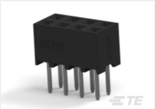
TE 产品编号 2307782-8 8P,2MM,B-B,REC,DRVT,2.0,0.38AU,TR,W/CAP
