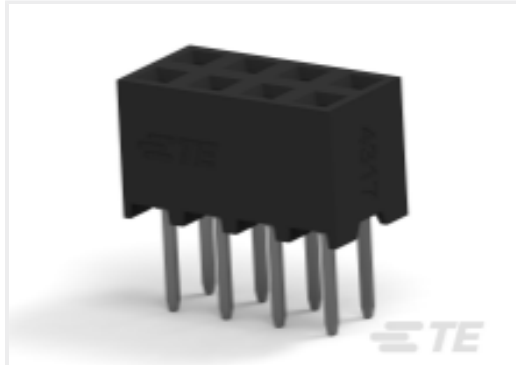
TE 产品编号 2314813-8 8P,2MM,B-B,REC,DRVT,2.0,0.38AU,TB,W/CAP
