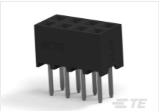
TE 产品编号 2307784-8 8P,2MM,B-B,REC,DRVT,3.2,0.38AU,TUBE
