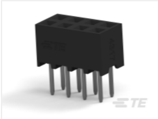
TE 产品编号 2314820-8 8P,2MM,B-B,REC,DRVT,2.7,0.1AU,TB
