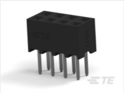
TE 产品编号 2307779-8 8P,2MM,B-B,REC,DRVT,2.0,0.1AU,TR,W/CAP
