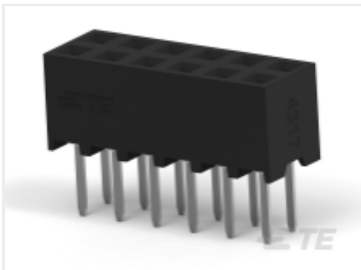
TE 产品编号 1-2307778-2 12P,2MM,B-B,REC,DRV,T,3.2,SN,TUBE
