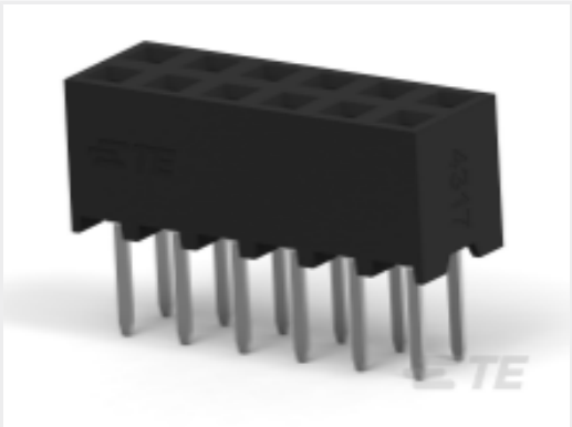
TE 产品编号 1-2307777-2 12P,2MM,B-B,REC,DRV,T,2.7,SN,TR,W /CAP
