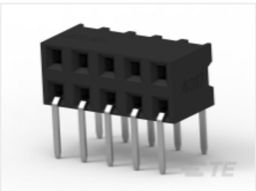
TE 产品编号 1-2314923-2 12P,2MM,B-B,REC,DRHZ,2.8,SN,TR
