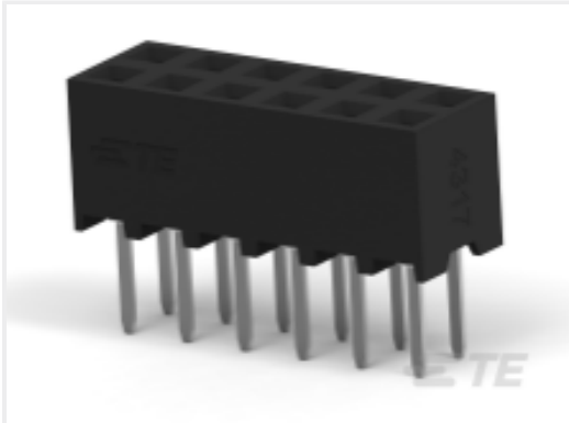
TE 产品编号 1-2314819-2 12P,2MM,B-B,REC,DRV,T,2.7,SN,TB
