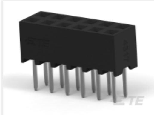
TE 产品编号 1-2314823-2 12P,2MM,B-B,REC,DRV,T,2.7,SN,TB W /CAP
