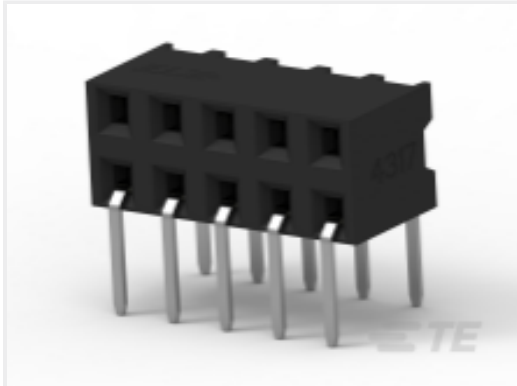
TE 产品编号 1-2314915-2 12P,2MM,B-B,REC,DRHZ,2.1,SN,TB
