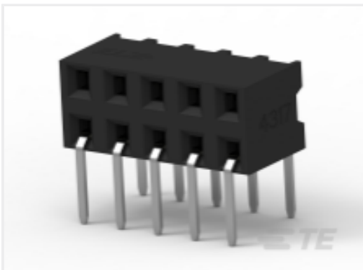
TE 产品编号 1-2307712-2 12P,2MM,B-B,REC,DRHZ,2.1,SN,TR
