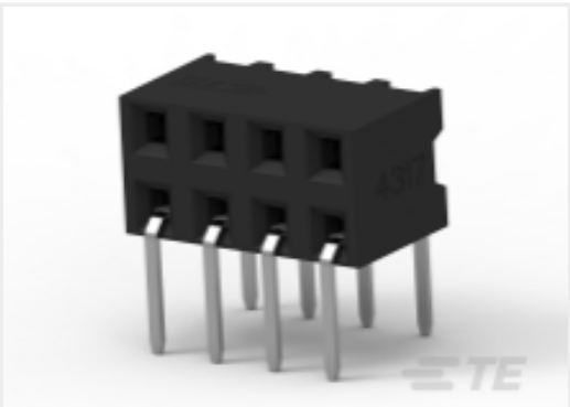
TE 产品编号 2307722-8 8P,2MM,B-B,REC,DRHZ,2.8,0.76AU,TB
