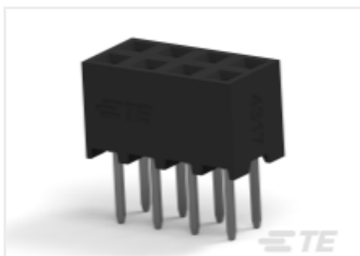
TE 产品编号 2307786-8 8P,2MM,B-B,REC,DRV,T,2.7,0.76AU,TR, W/CAP
