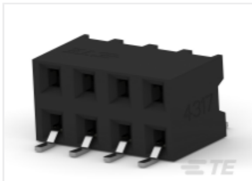
TE 产品编号 2314942-8 8P,2MM,B-B,REC,DRHZ,SMD,0.76AU, TB
