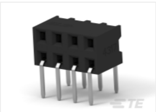
TE 产品编号 2314926-8 8P,2MM,B-B,REC,DRHZ,2.8,0.76AU,TR
