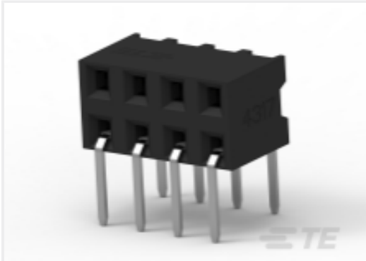
TE 产品编号 2307721-8 8P,2MM,B-B,REC,DRHZ,2.1,0.76AU,TR
