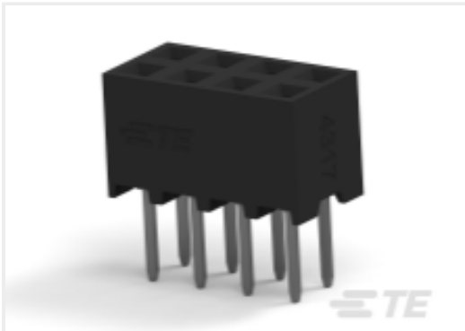
TE 产品编号 2314814-8 8P,2MM,B-B,REC,DRV,T,2.0,0.76AU,TB, W/CAP
