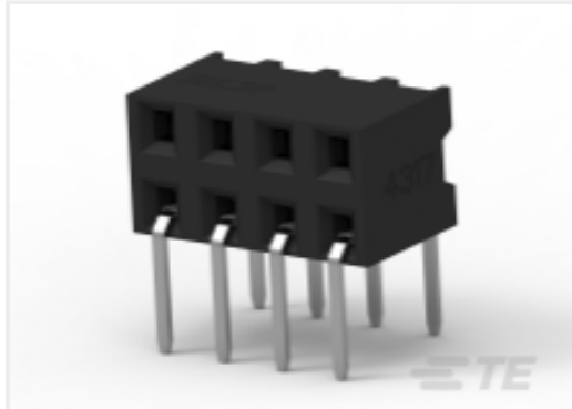
TE 产品编号 2307723-8 8P,2MM,B-B,REC,DRHZ,3.4,0.76AU, TUBE
