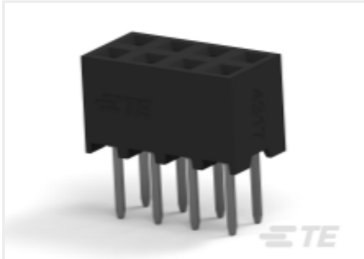
TE 产品编号 2307787-8 8P,2MM,B-B,REC,DRV,T,3.2,0.76AU, TUBE
