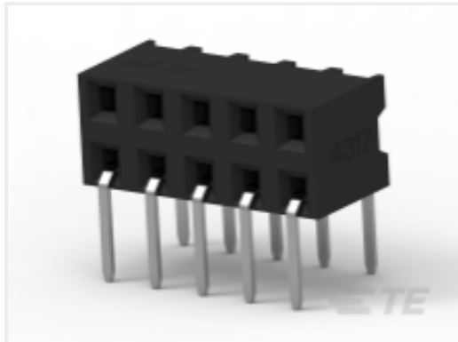
TE 产品编号 1-2307718-4 14P,2MM,B-B,REC,DRHZ,2.1,0.38AU,TR
