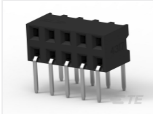
TE 产品编号 1-2307719-4 14P,2MM,B-B,REC,DRHZ,2.8,0.38AU,TB
