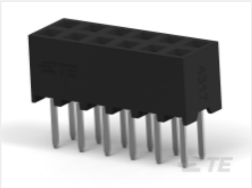
TE 产品编号 1-2307784-4 14P,2MM,B-B,REC,DRV,T,3.2,0.38AU,TUBE
