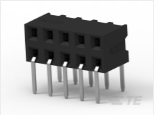
TE 产品编号 1-2314917-4 14P,2MM,B-B,REC,DRHZ,2.1,0.38AU,TB
