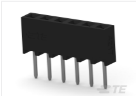
TE 产品编号 2314869-6 6P,2MM,BB,REC,SRVT,2.0,0.38AU,TB,W/CAP
