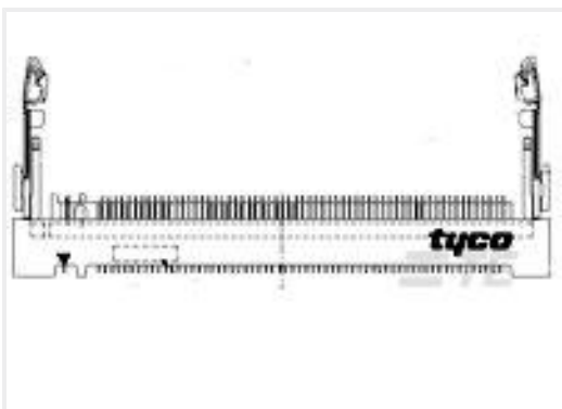
TE 产品编号1717831-1 MINI PCI EXPRESS SEMI HARD TRAY CONN
