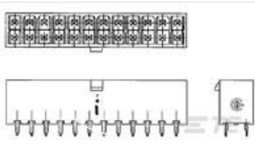
TE 产品编号2-1586037-4 24P VERT HDR VAL-U-LOK V2
