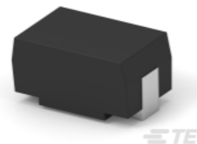
TE 产品编号2-1879233-5 SMD 功率电阻器: 7 瓦特, .10-500 欧姆
