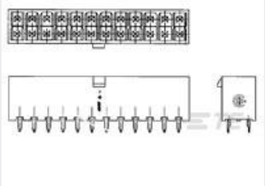
TE 产品编号1-1586038-0 10P VRT HDR VAL-U-LOK V0
