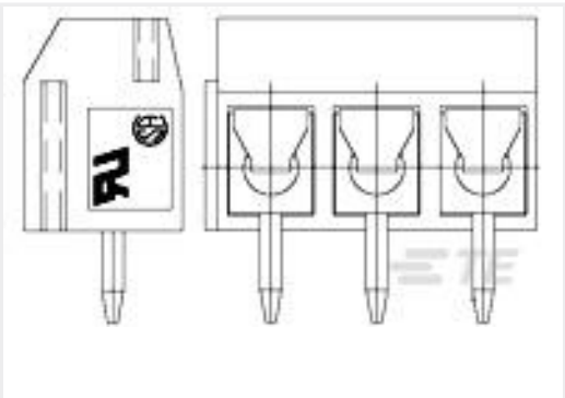
TE 产品编号1776244-3 3P TB ,90deg, VT, 5mm, Blue,w /interlock
