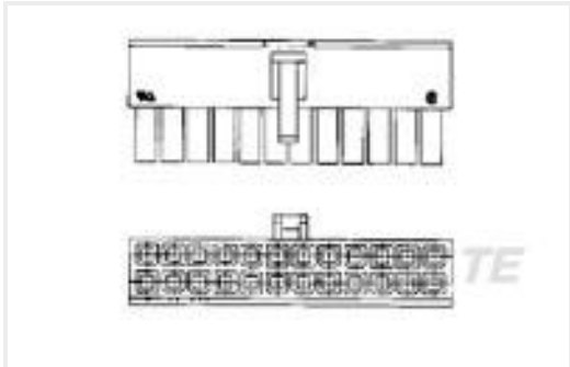
TE 产品编号794954-4 4P RCPT VAL-U-LOK V2
