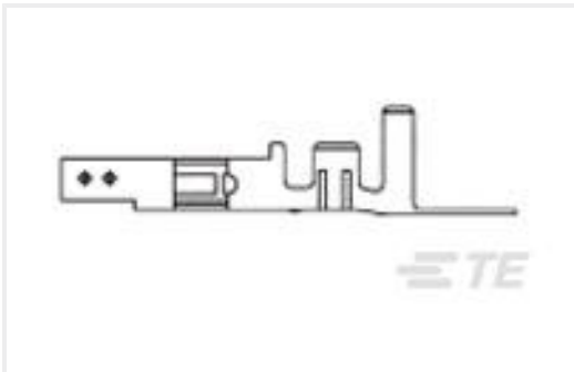
TE 产品编号794956-1 VAL-U-LOK SKT BR SN 22-18AWG
