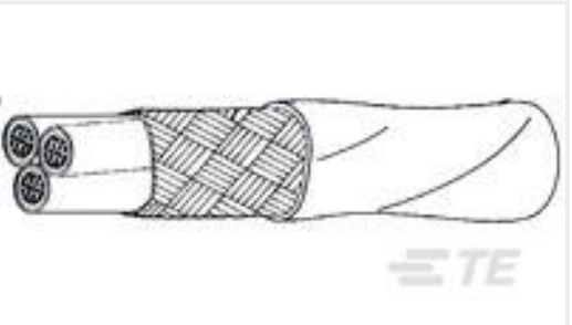
TE 产品编号201097-1 MIN PIN
