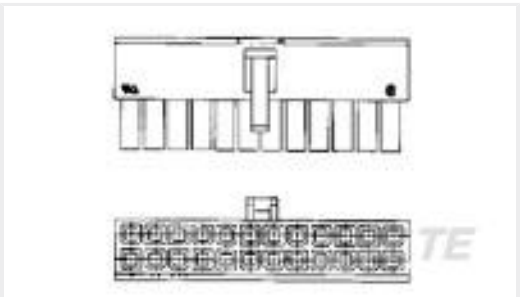
TE 产品编号2-1586765-0 20P RCPT VAL-U-LOK GW
