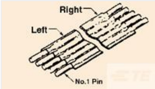
TE 产品编号6-1437187-4 FST-22A-18
